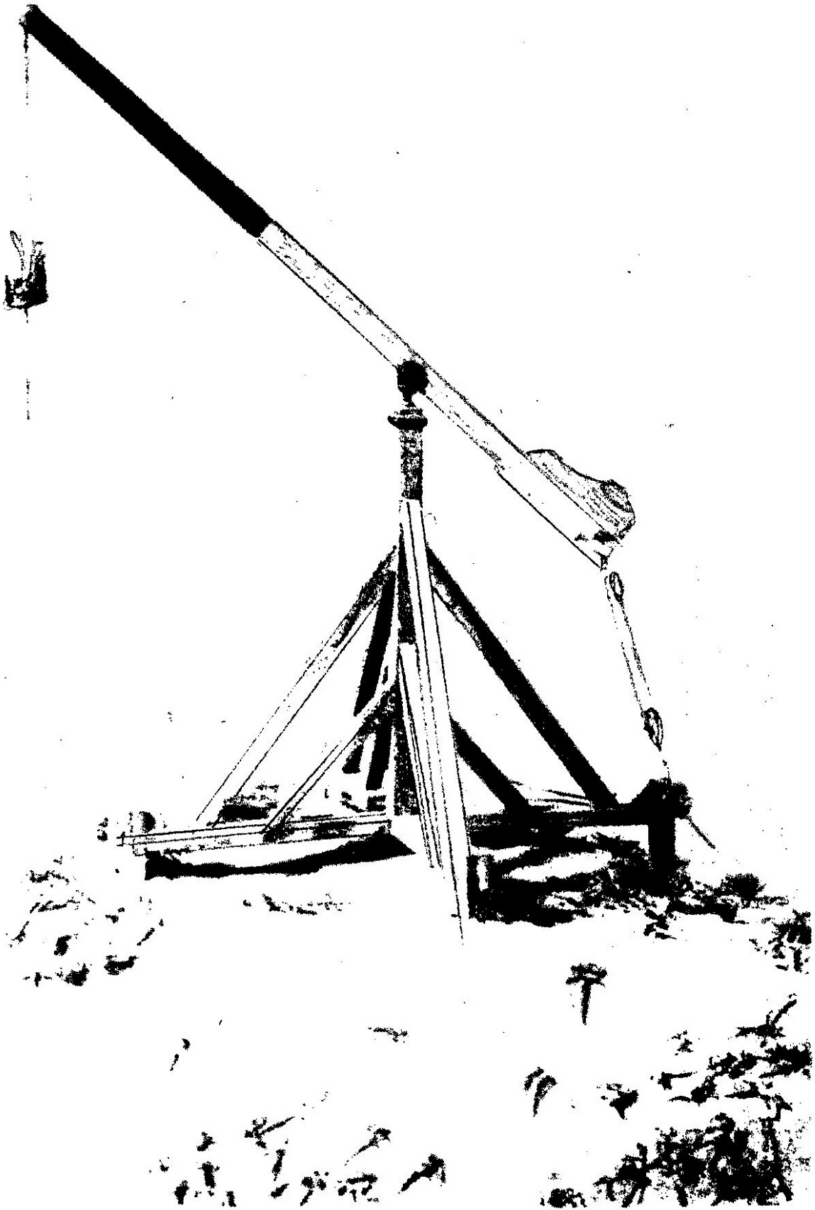
Anholt vippefyр 1708. Vippefyrene blev konstrueret 1626 af Jens Pedersen Grove og opsattes i klitterne på Skagen, Anholt, Falsterbo m. fl. steder. Model i skala 1:50.
